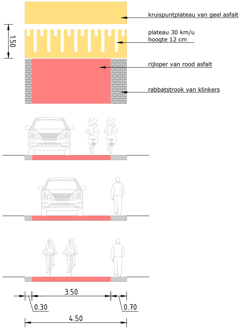
Principeprofiel SCHAAL 1 : 300
