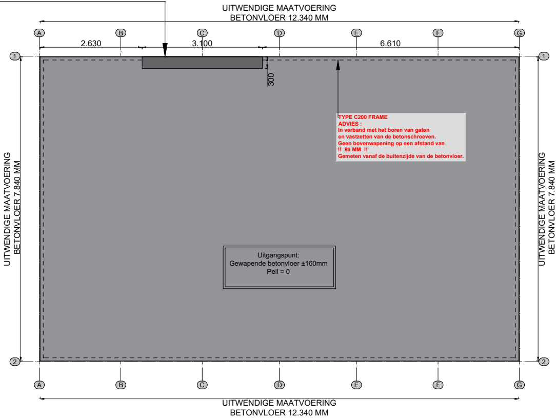
BETONTEKENING
