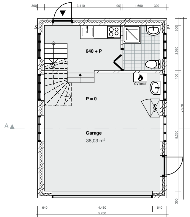
Begane grond GO: 38,03 m2
