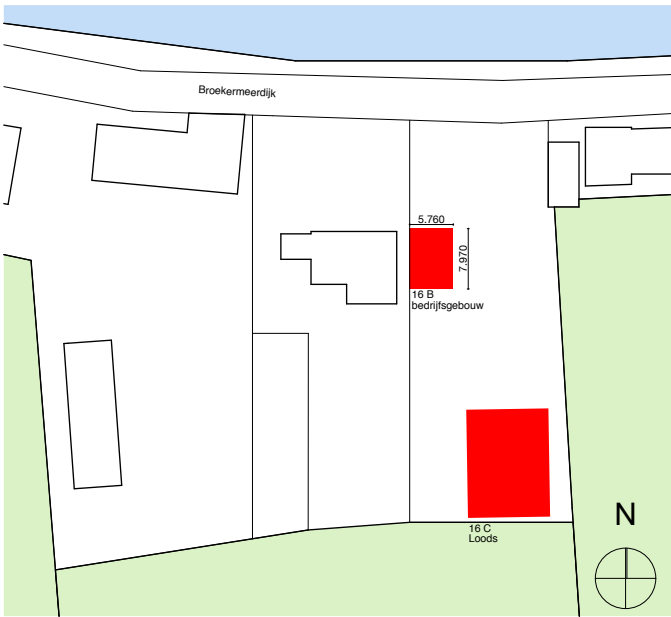
Situatie 1:1000
