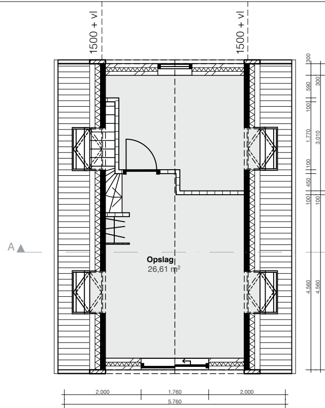
1ste verdieping GO: 26,61 m2
