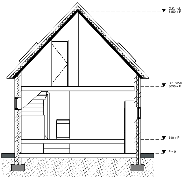
Doorsnede A - A
