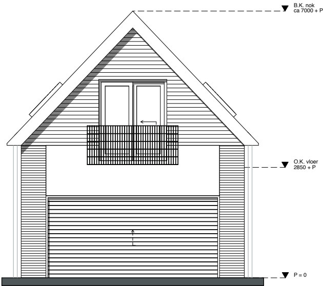
Achtergevel
