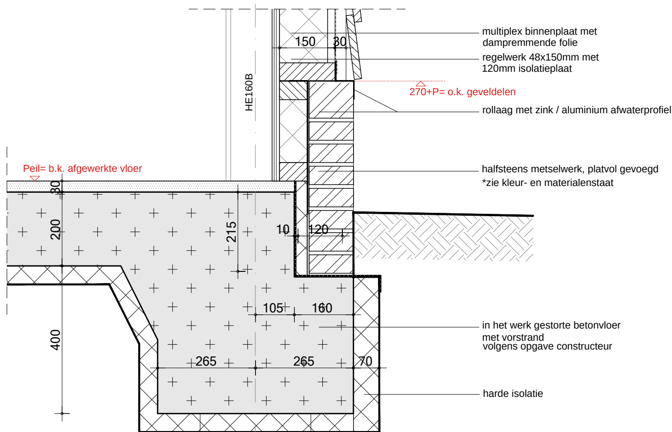
DETAIL V01 FUNDERING AANSLUITING
