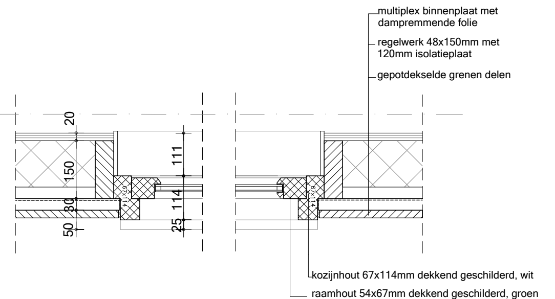
DETAIL H01 KOZIJN AANSLUITING
